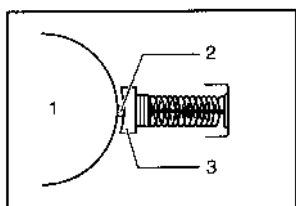
1. Kommutátor; 2. Szigetelőcsűcs; 3. Szénkefe
