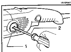
1. Kefetartó rögzítősapkája 2. Csavarhűző
