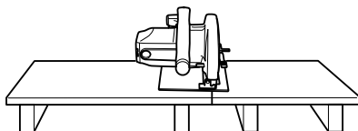
Podepřením desky nebo panelu v blízkosti řezu zamezíte zpětnému rázu.
