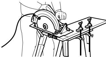
Typické zobrazenie správneho opretia ruky, podopretia obrobku a vedenia napájacieho prívodu (ak je to použiteľné).
