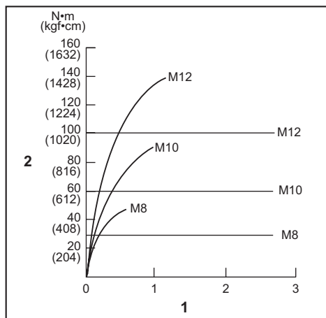
1. Doba utahování (sekundy) 2. Utahovací moment
